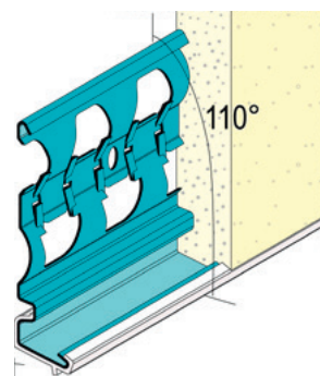
Abb. 4 Putzabschluss-/Sockelprofil.
